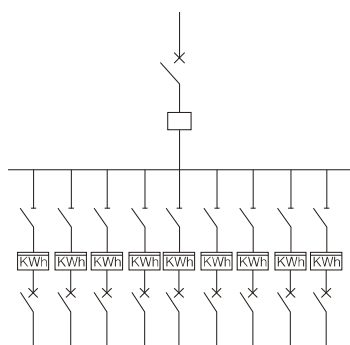
图1 接线图
